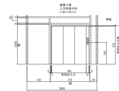
出入口正面図
